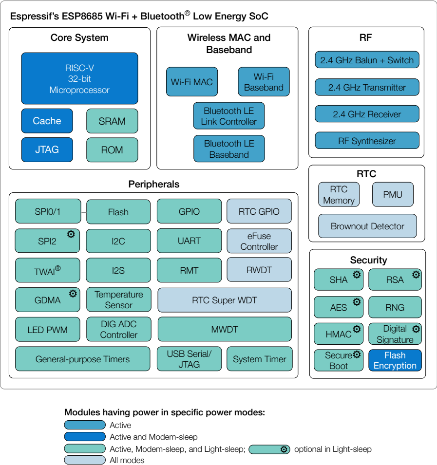
ESP8685 功能框图
