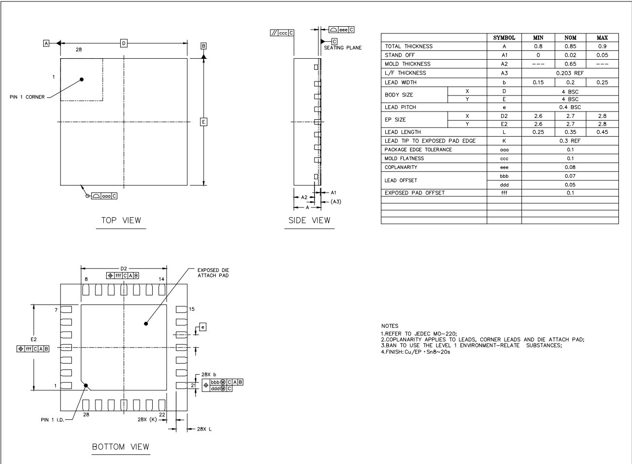
图 6-1. QFN28 (4x4 mm) 封装
