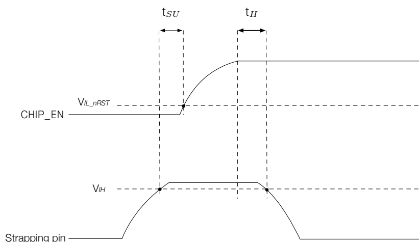
图 2-1. Strapping 管脚的时序参数图
