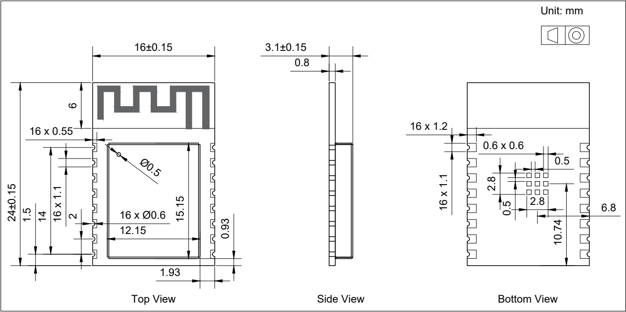
图 6: 模组尺寸
