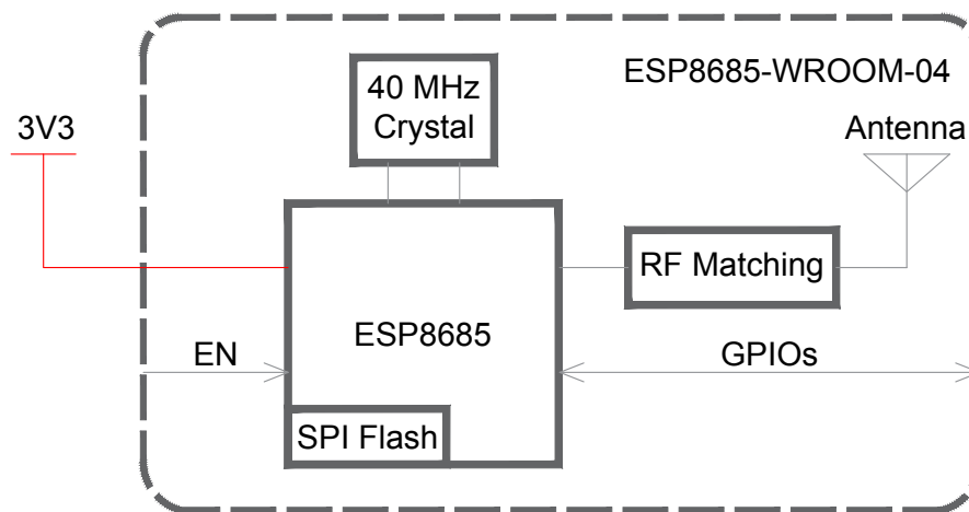
图 1: 功能框图
