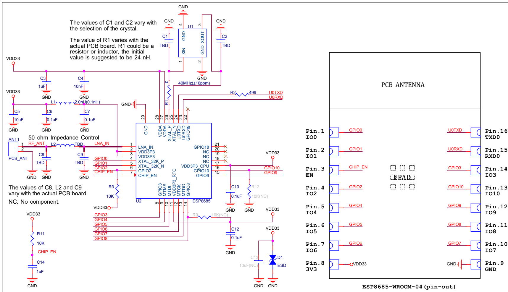
图 4: 原理图
