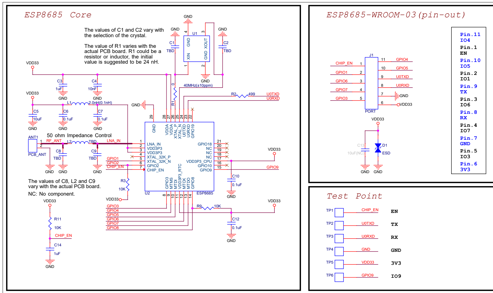
图 4: 原理图
