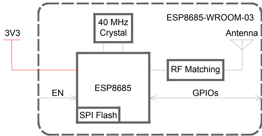
图 1: 功能框图
