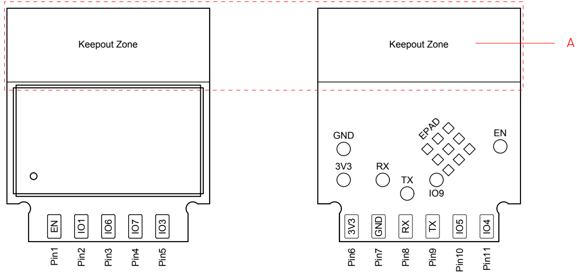
图 2: 管脚布局（顶视图和底视图）
