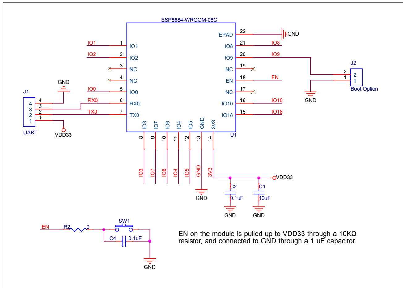
图 5: 外围设计原理图
