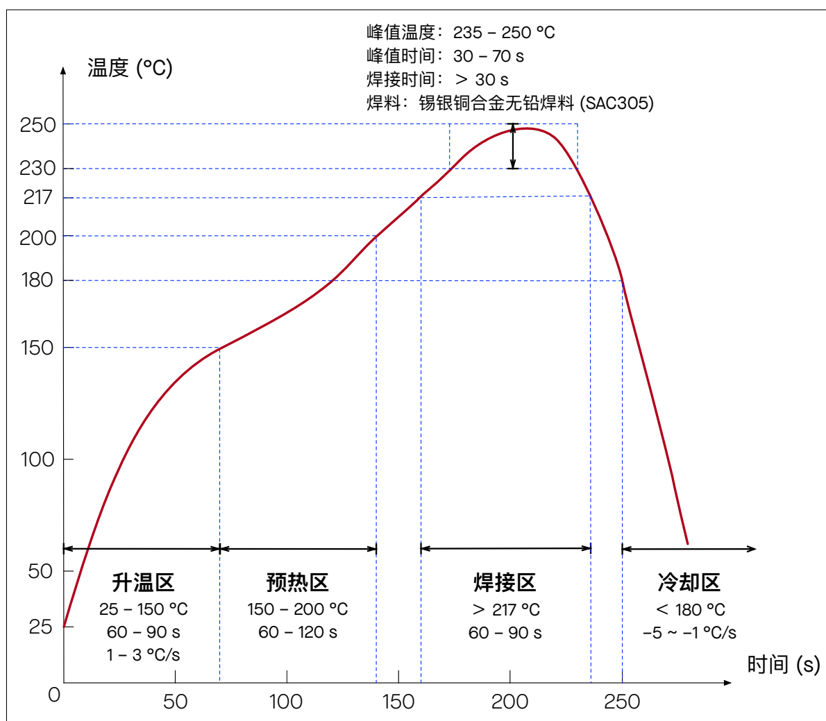
图 9: 回流焊温度曲线
