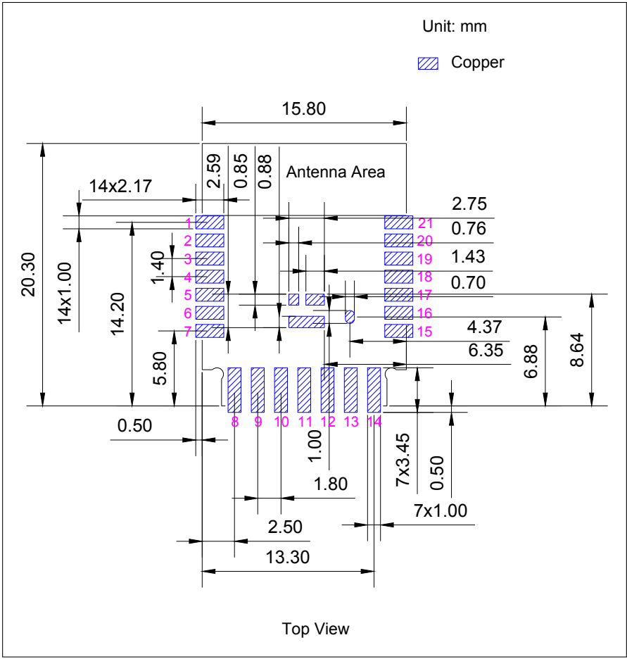
图 7: 模组表面贴装推荐 PCB 封装图形
