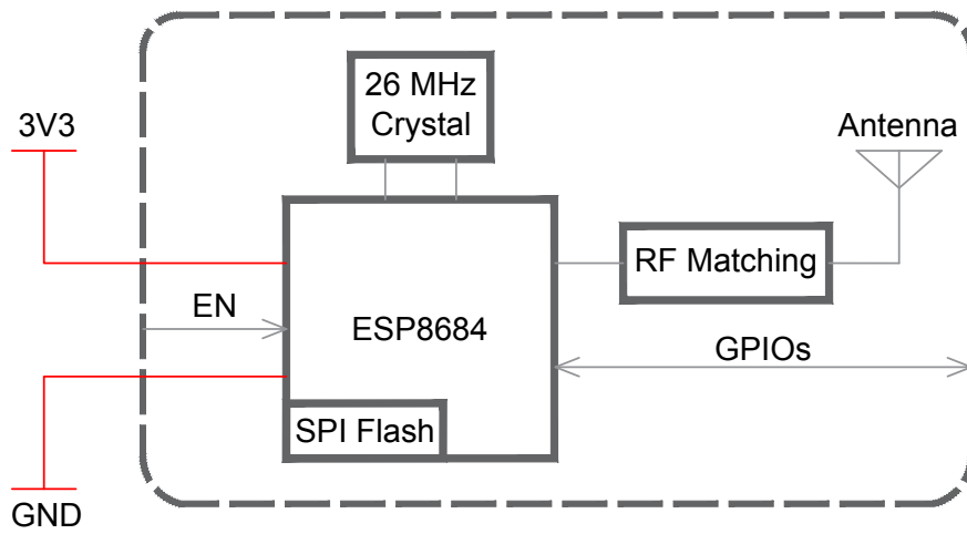
图 1: ESP8684-WROOM-06C 功能框图
