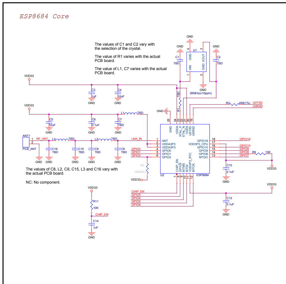
图 4: ESP8684-WROOM-06C 原理图
