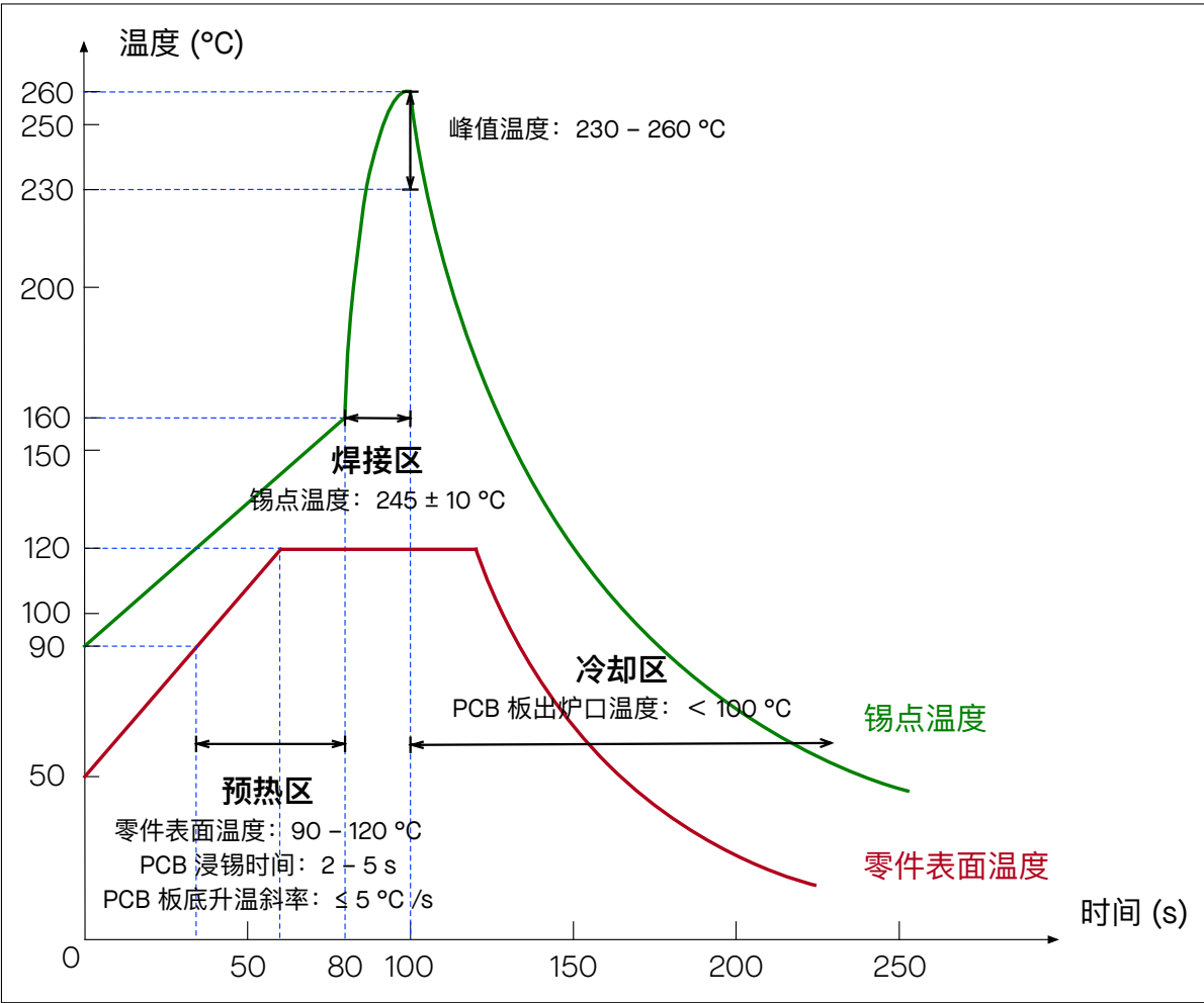
图 10: 波峰焊温度曲线
