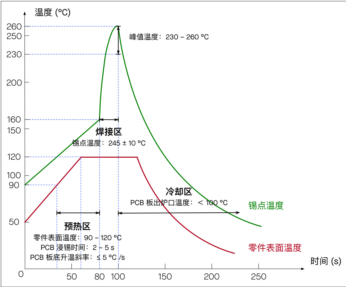
图 9: 波峰焊温度曲线
