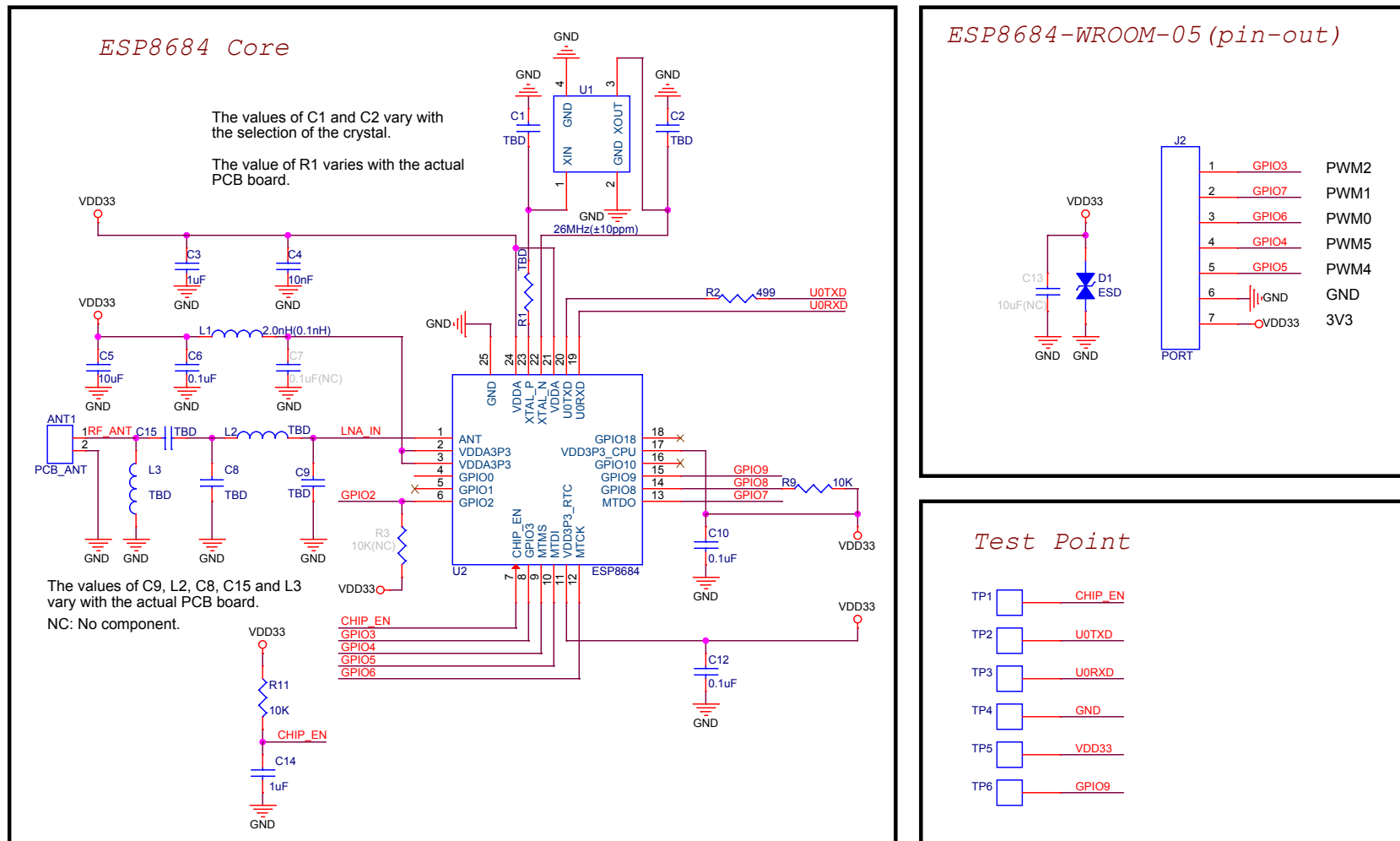
图 4: ESP8684-WROOM-05 原理图
