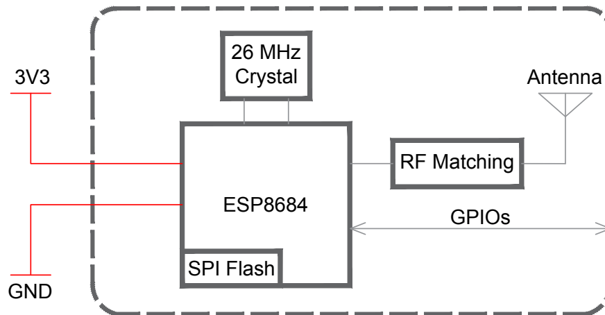
图 1: ESP8684-WROOM-05 功能框图
