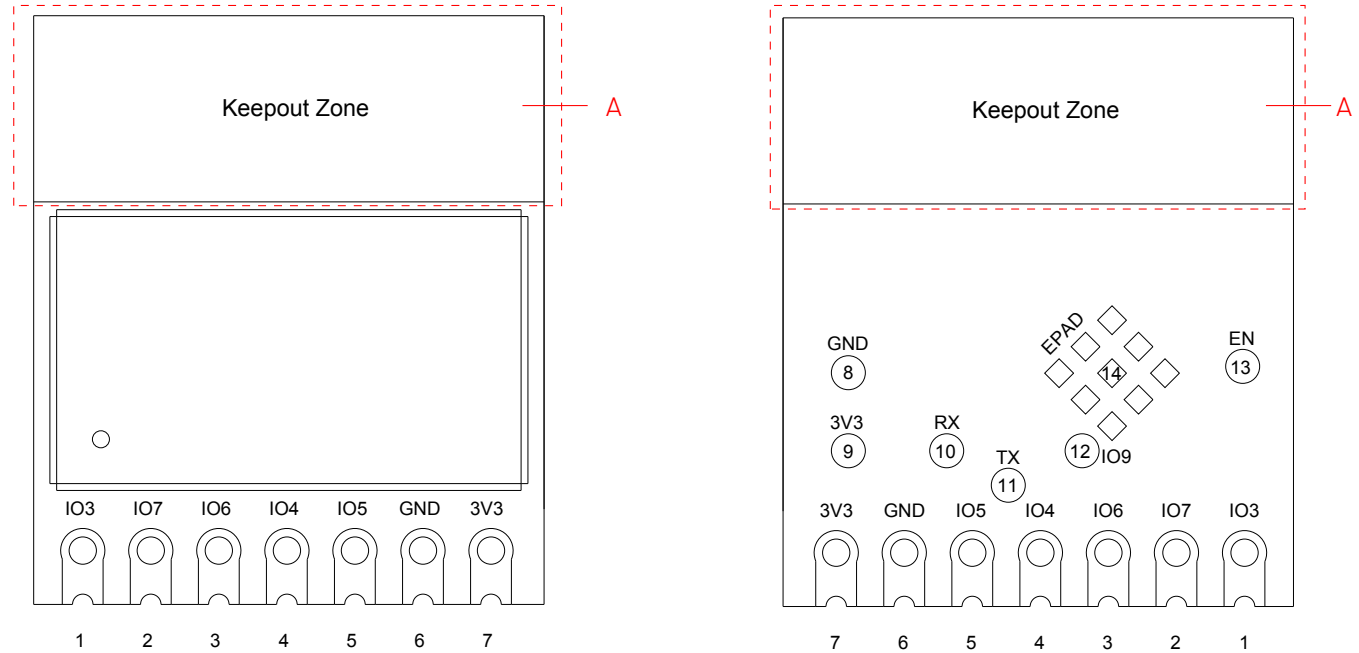
图 2: 管脚布局（顶视图和底视图）
