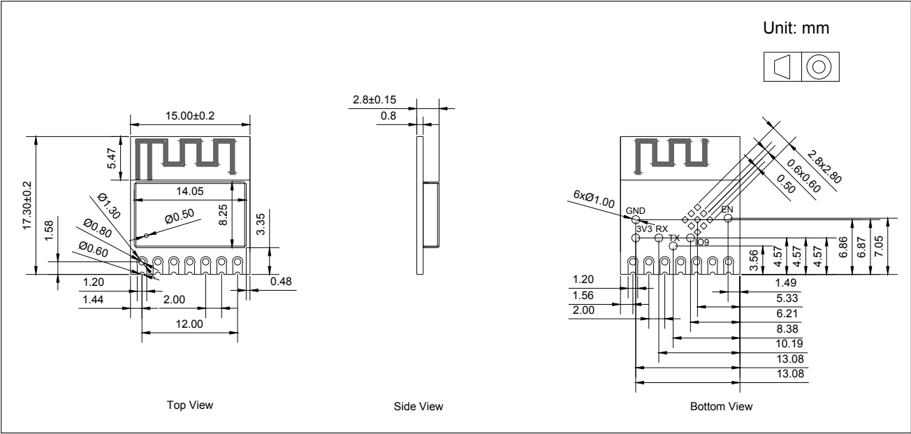
图 6: 模组尺寸
