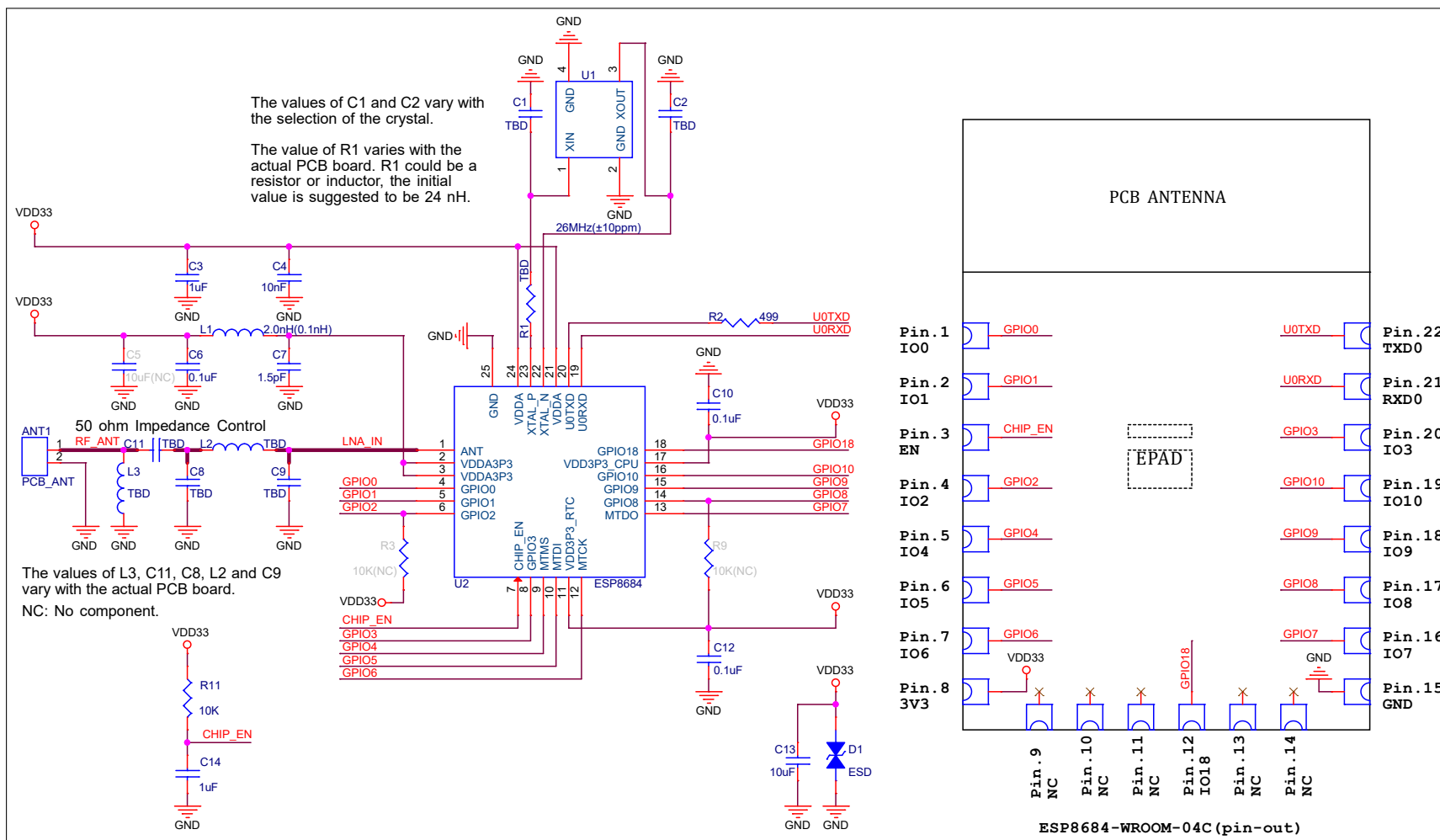
图 4: ESP8684-WROOM-04C 原理图
