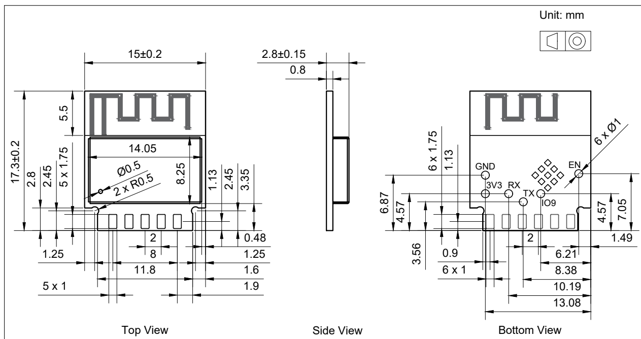
图 6: 模组尺寸
