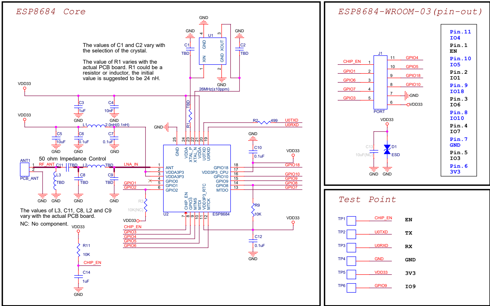
图 4: ESP8684-WROOM-03 原理图
