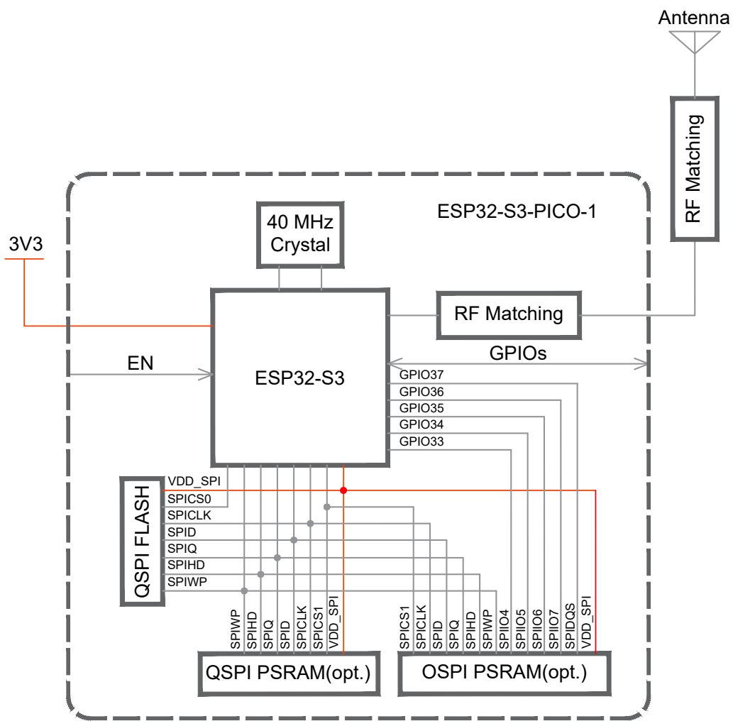
ESP32-S3-PICO-1 功能框图
