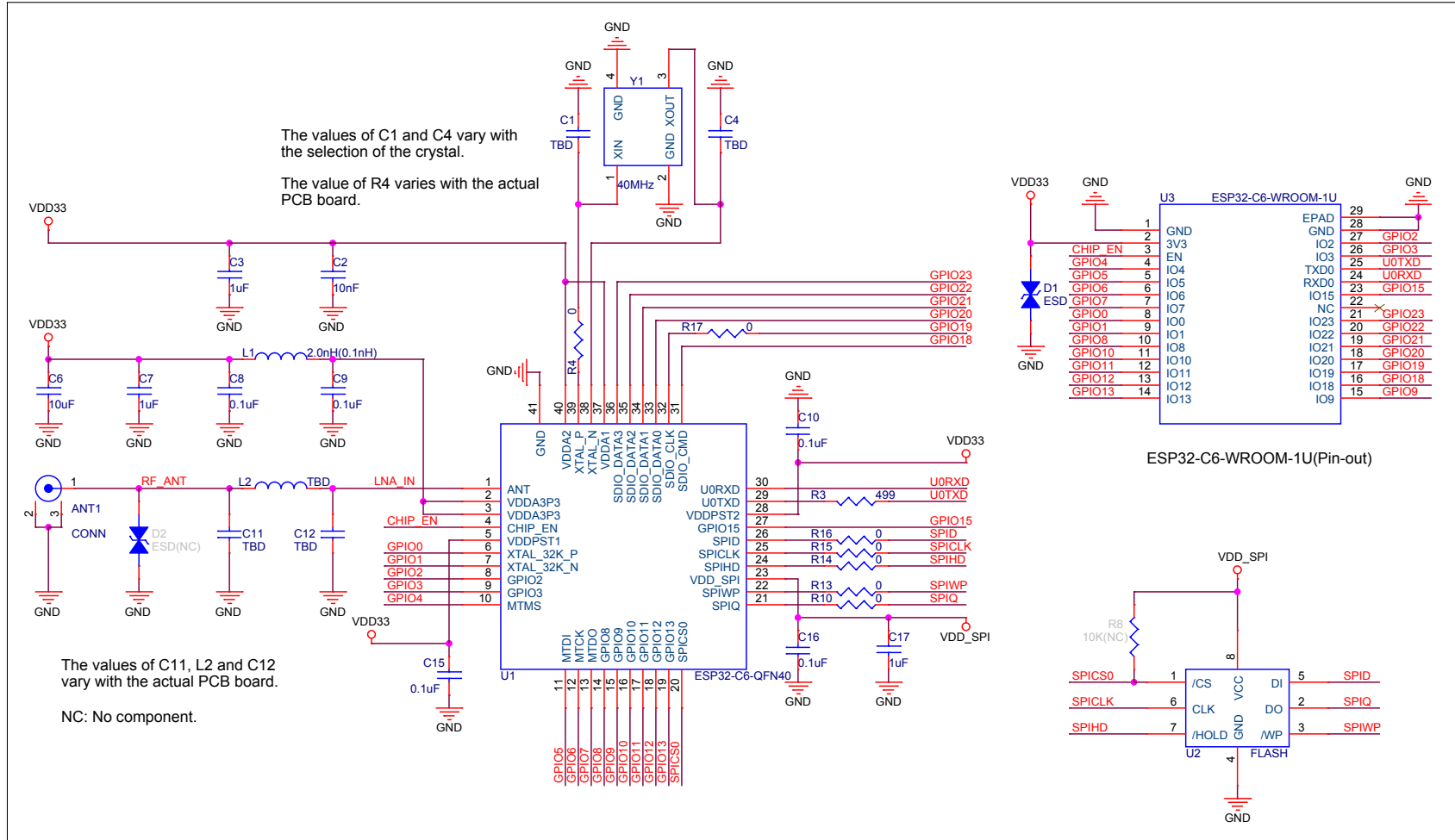
图 6: ESP32-C6-WROOM-1U 原理图
